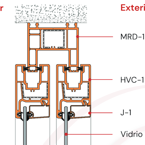
Det. 04
