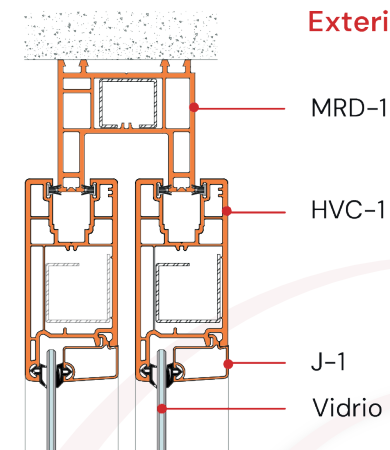
Det. 04
