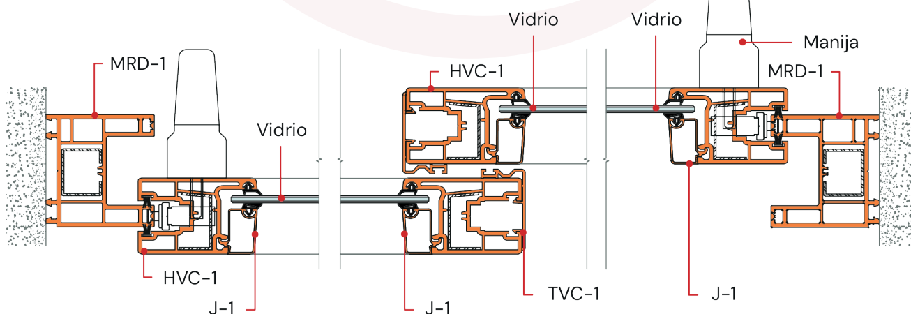
Det. 01
