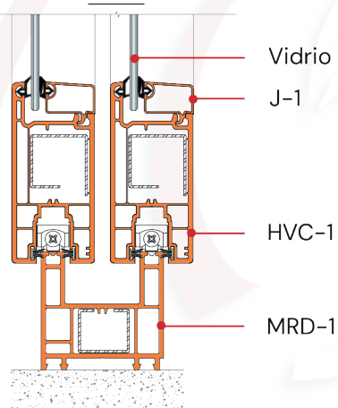
Det. 05
