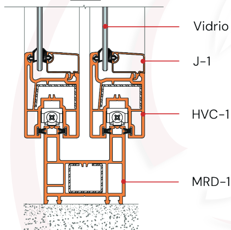
Det. 05
